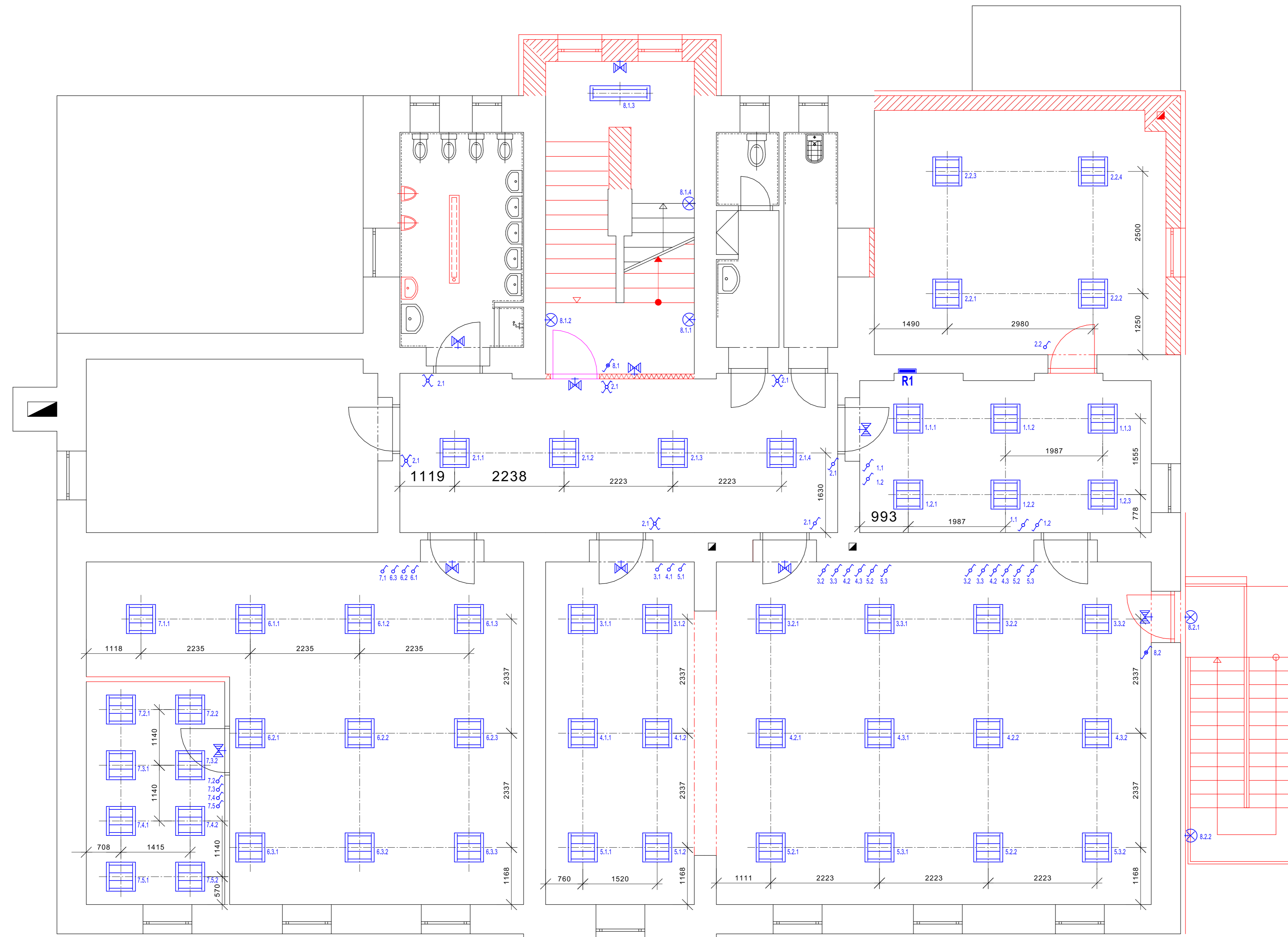
PŮDORYS 2. NP - MŠ
